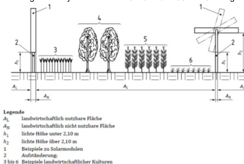
Abb. 1: Agrar-PV-System nach DIN 91434:2021-05 SPEC Kategorie II, Var. 2
