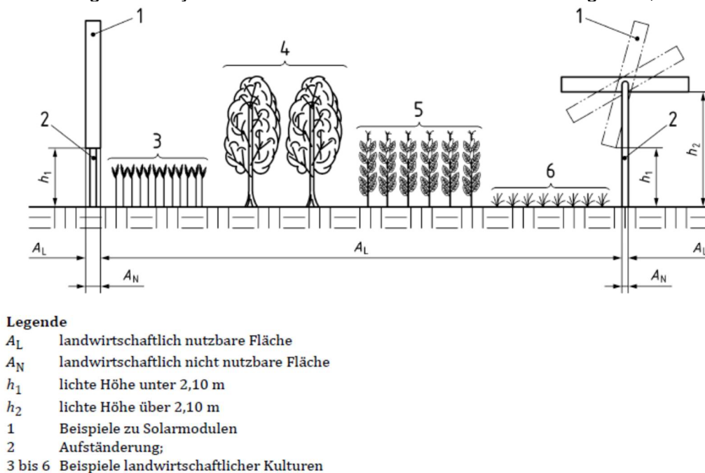
Abb.: 1 – Agrar-PV-System nach DIN 91434: 2021-05 SPEC Kategorie II, Var. 2
